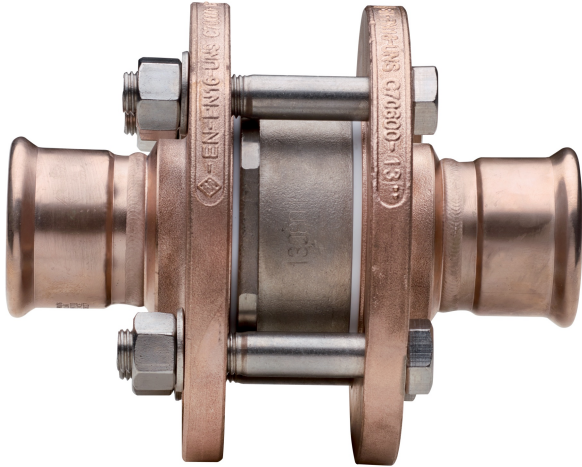
Valvula de retencion à disco PN16.
